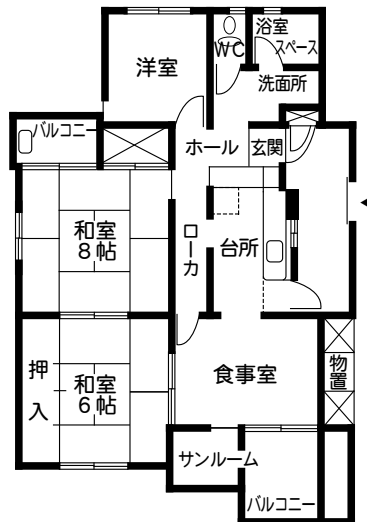
庄西 1 号棟 (74.70㎡)
