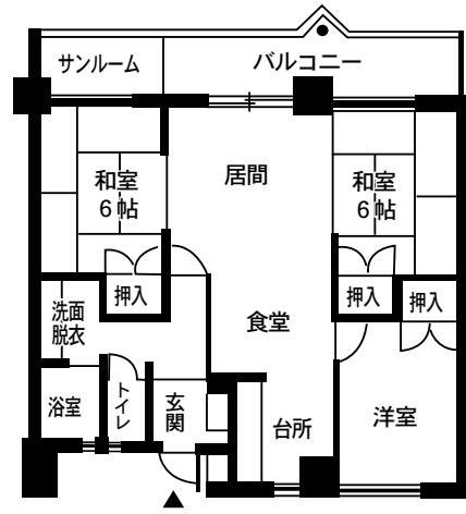
立町 A-1 妻 (83.67㎡)
